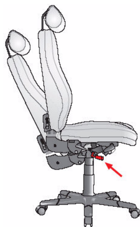
Wippmechanik Hebel nach vorne drehen: fixiert Hebel nach hinten drehen: freie Bewegung
