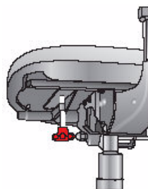
Feineinstellung mit Handrad Wippwiderstand individuell anpassbar
