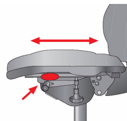
Sitztiefenverstellung Knopf hineindrücken, Sitz vor- oder zurückschieben. Knopf loslassen fixiert
